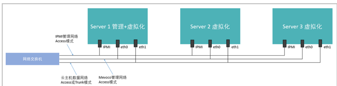
图 2: ZStack本地存储方案网络拓扑图
