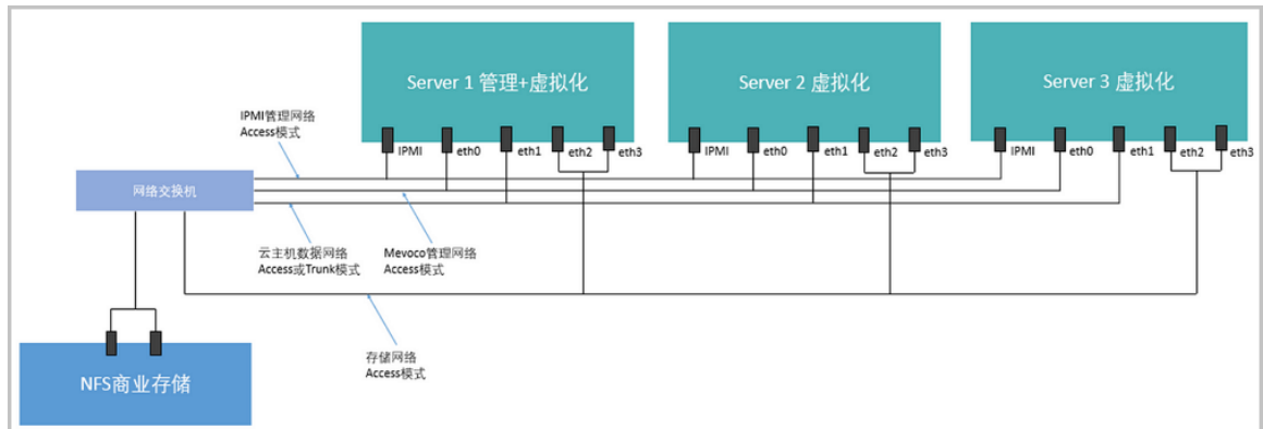
图 4: ZStack NFS商业存储方案网络拓扑图
